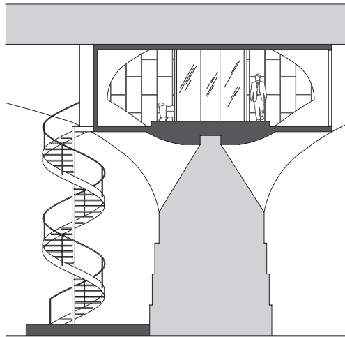
Sektion BB
