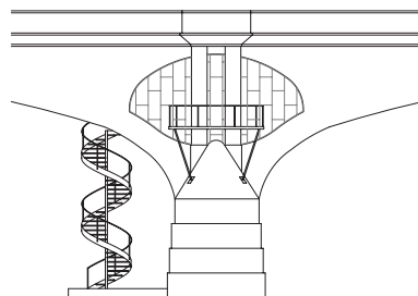
Västra fasaden
